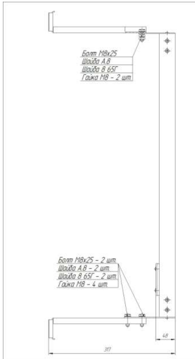
Рисунок 3. Крепления (в комплекте)
