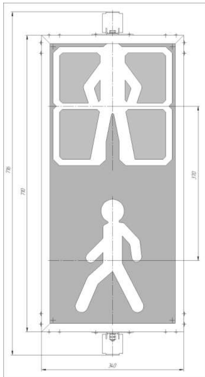
Рисунок 1. Светофор пешеходный СПО-300
